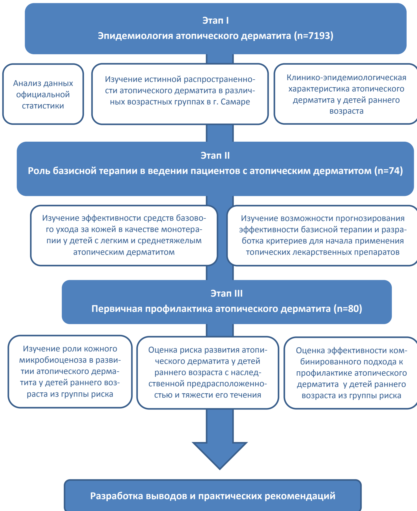
Рисунок 1. Дизайн исследования.
