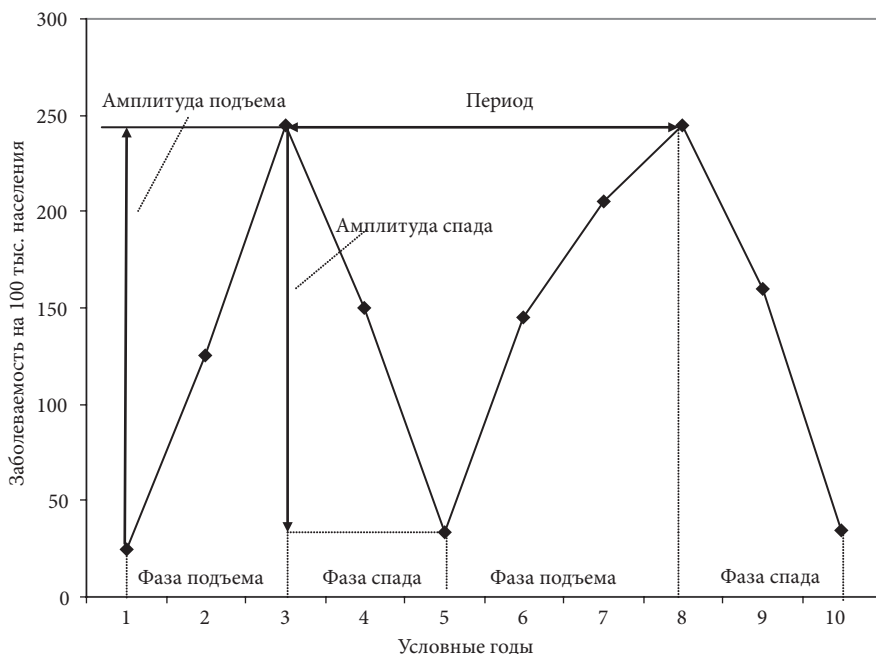
Рис. 1.7. Циклические колебания с периодом 5 лет (первый цикл — годы 1, 2, 3, 4, 5; второй цикл — 6, 7, 8, 9, 10; годы подъема (максимального) — 3, 8; годы спада (максимального) — 1, 5, 10)
