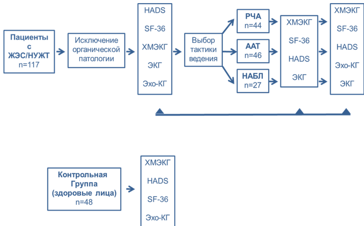
Рисунок 1 – Дизайн исследования
