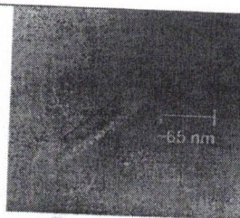
Бактериофаг λ
