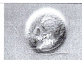
Хламидомонада ( Chlamydomonas reinhardtii )
