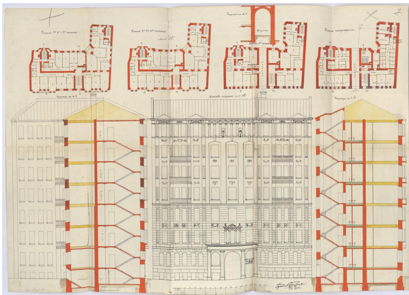
Рисунок 9 – Проект 7-этажного здания для зубоврачебной школы И.М. Коварского. 1905 год.
