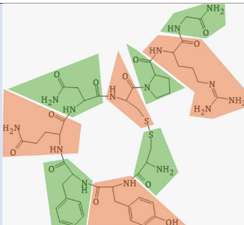
Вазопрессин
