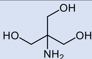
Трис (триметамин)
