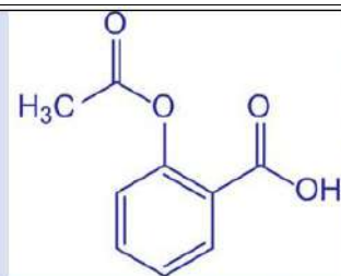
Аспирин
