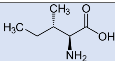
Изолейцин
